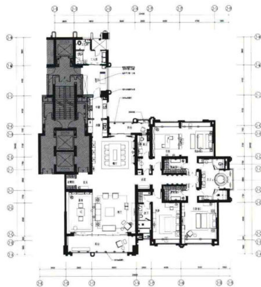
平面布置图
