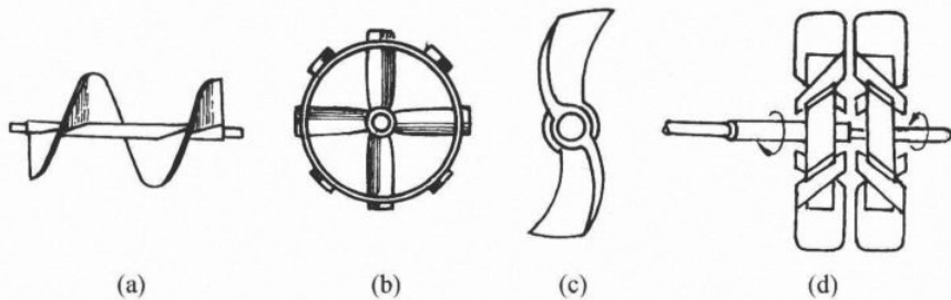
图 1-2 早期螺旋推进器的几种形式
