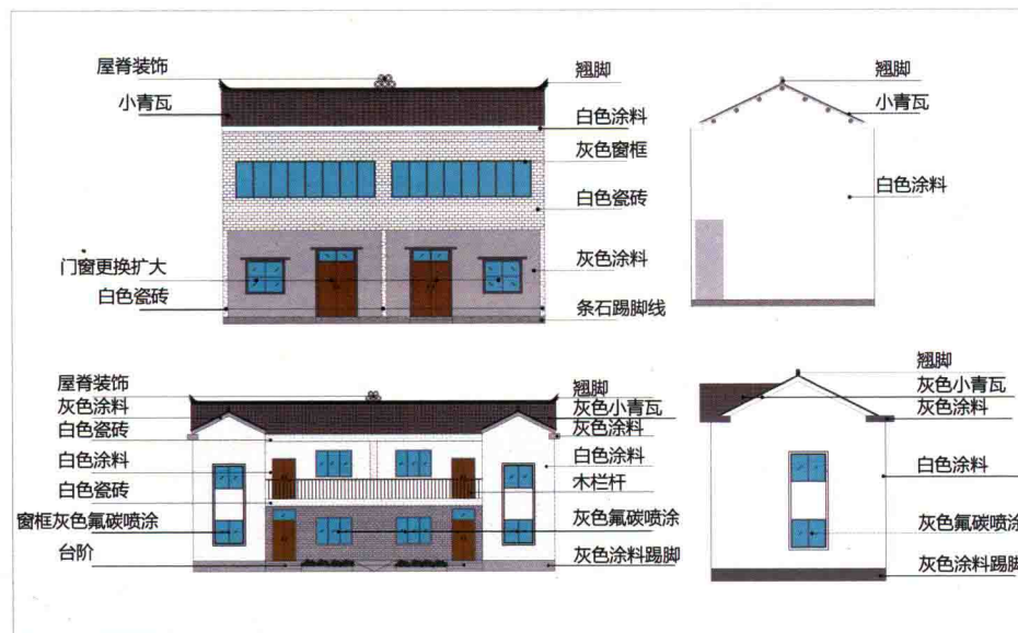
建筑改造技术导则
