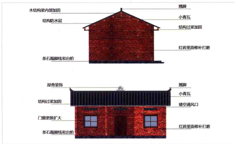
建筑改造技术导则 (一)
