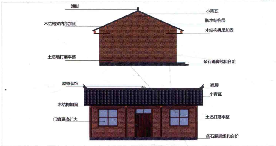
建筑改造技术导则 (二)
