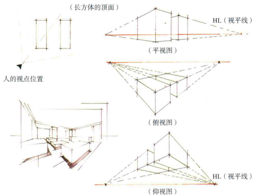
图 1-28 两点透视
