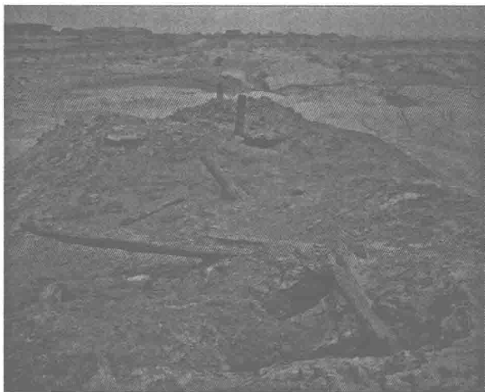
图9 “居卢营仓”仓址
