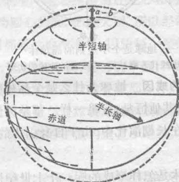
地球椭球体
