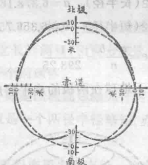
地球是个不规则的椭球体 虚线代表椭球体,实线表示地球的实形
