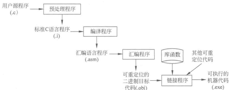
图 1.4 C 语言编译过程
