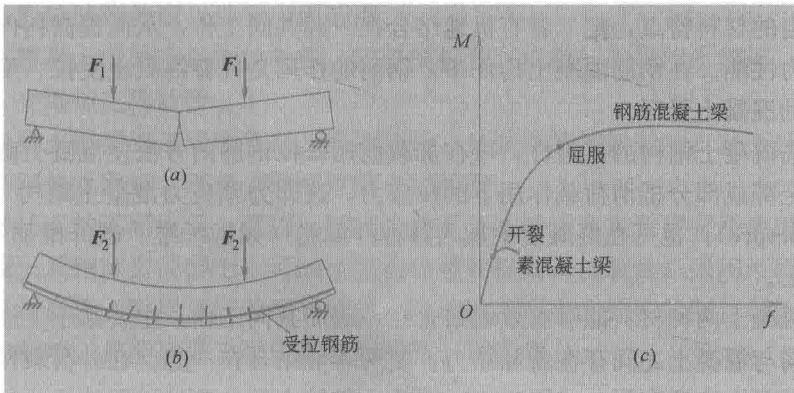
图 1-1 素混凝土梁及钢筋混凝土梁
