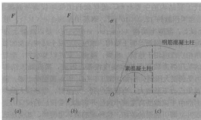
图 1-2 素混凝土与钢筋混凝土轴心受压构件
