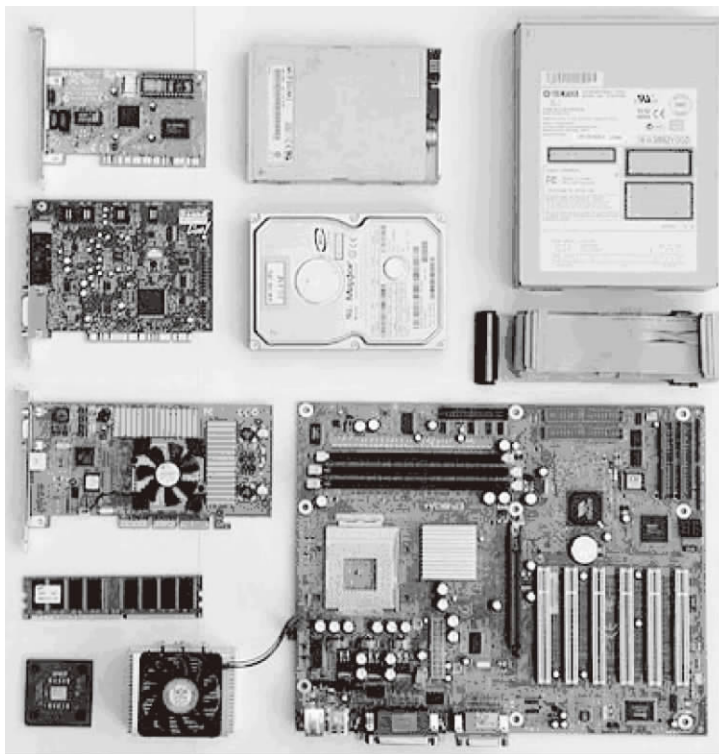
图 1-2 计算机硬件产品
