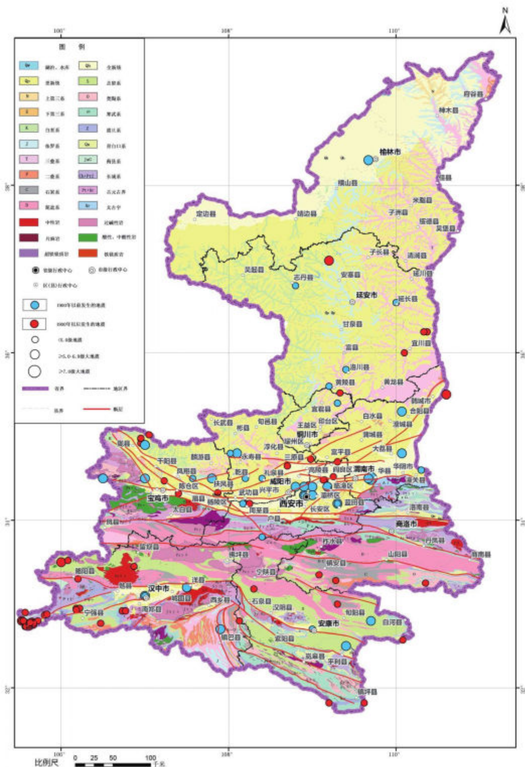
陕西省地震构造图
