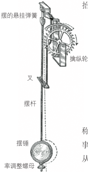
机械钟表一般由原动系、传动系、擒纵调速系、上条拨针系和指针系组成，工作原理基本相同，包括日历机构。最早的擒纵机构由英国人发明，18—19 世纪，钟表制造业逐步实现量产，并达到相当高的水平。图为出现在 1906 出版的物理书中的锚式擒纵摆图。
