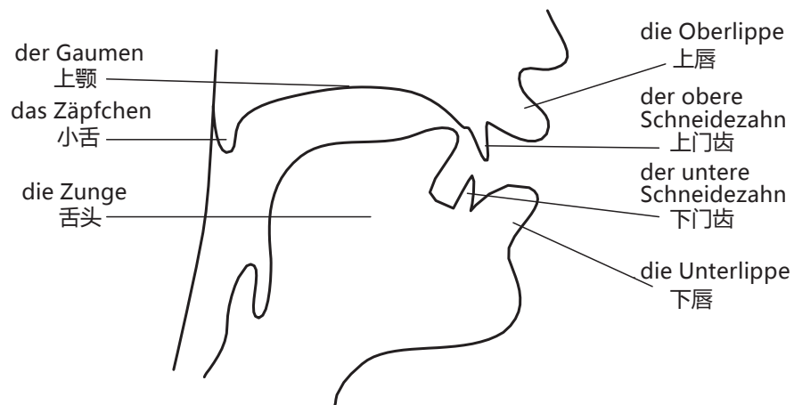
sch [ʃ] 在发音时的口腔截面图示
