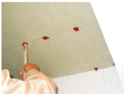
图1-51 涂刷防锈漆
