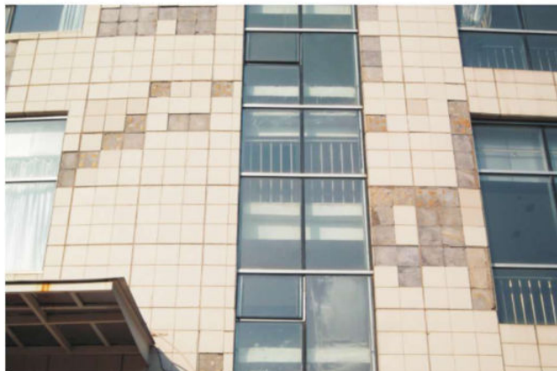
图1-27 墙面砖脱落
