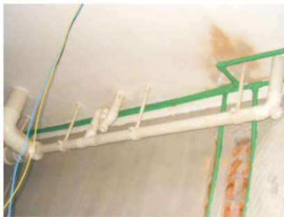
图1-50 排水管道
