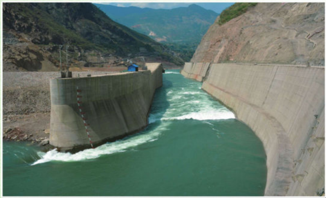
◆ 2017年1月23日，金沙水电站成功截流。图为导流明渠过水
