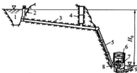
图 1-2 水电站发电原理
