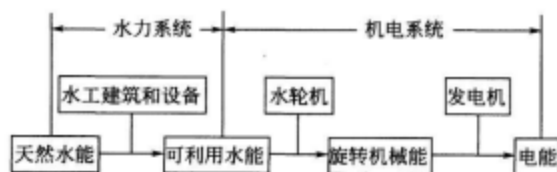
图 1-1 水力发电系统的组成
