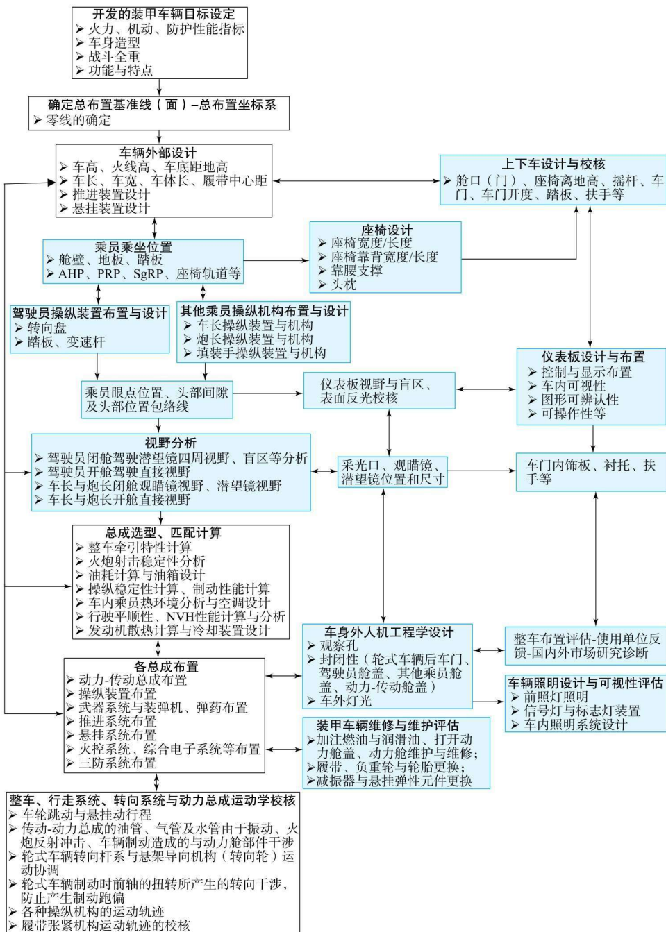
图 3.43 装甲车辆总布置与人机工程设计流程图
