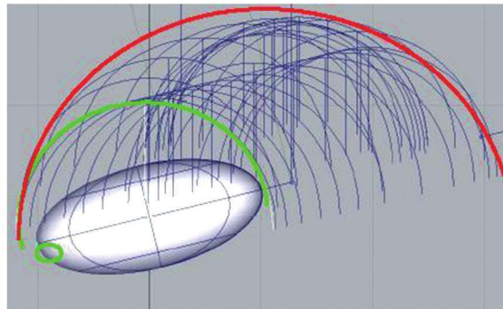
图 3.42 驾驶员头廓包络线（红线）和乘员头廓包络线（绿线）
