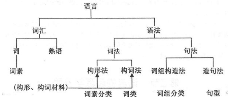
图 1-1 语言结构图
