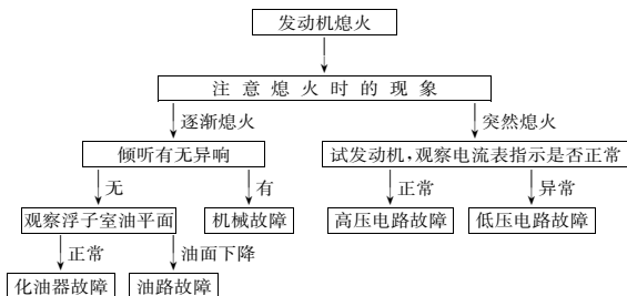
图 1-3 发动机熄火故障诊断流程图
