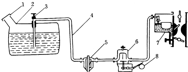
图 1-2 汽油机油路故障一般部位
