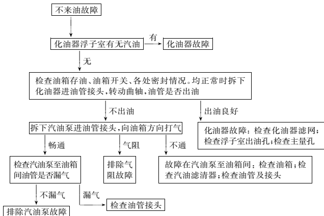
图 1-1 不来油故障诊断流程图
