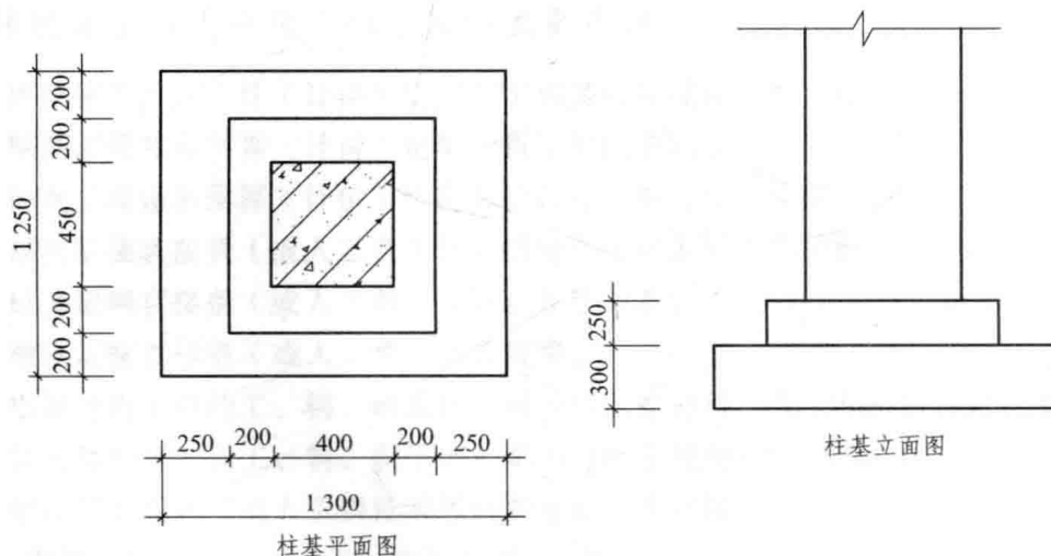
图 1.1 现浇独立基础
