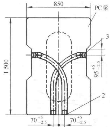
图 1-9 轨道梁电缆管道截面
