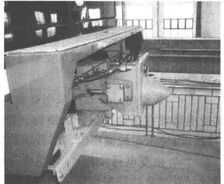
图 1-13 密接式车钩
