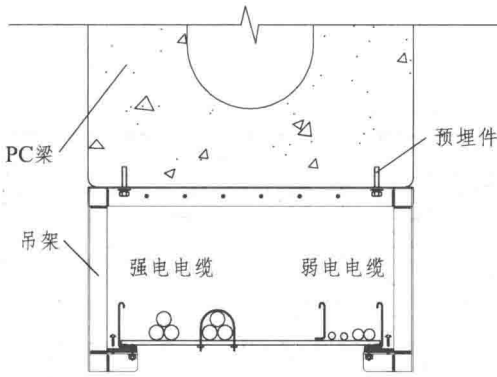
图 1-11 轨道梁下方吊架敷设 (重庆轨道二号线)
