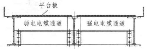
图 1-10 检修通道区间电缆敷设（重庆轨道三号线）
