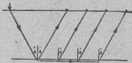
图 4 折射简图 (条件为 v_2 > v_1 )
