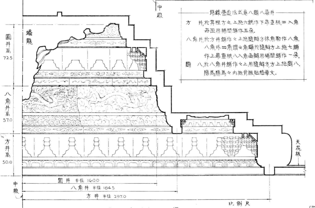
北平故宮太和殿龍井
