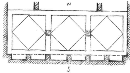
山東日照某漢墓平面仰視
