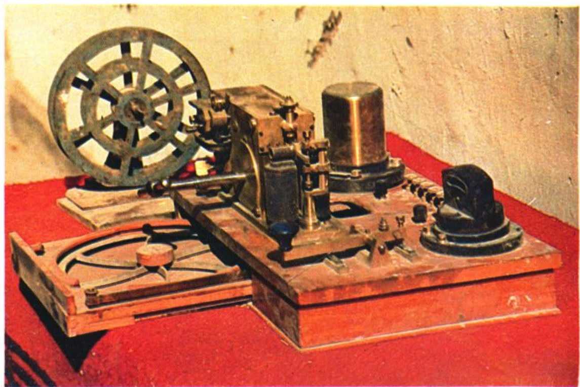
3、哈密电报局早期使用的莫尔斯收发报机
