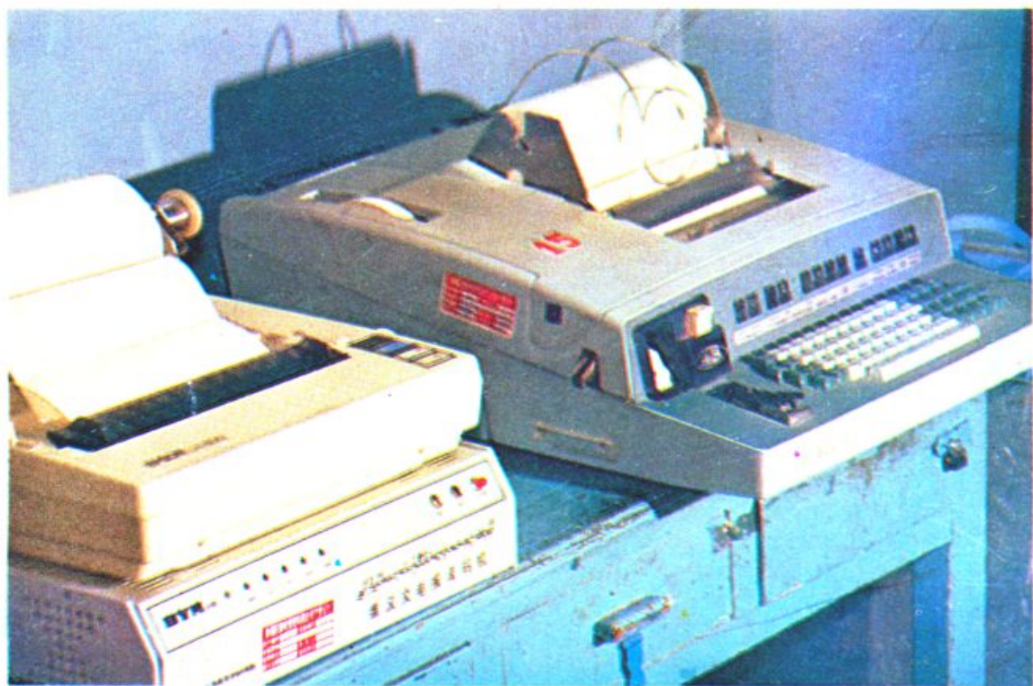
14、电报译电设备
