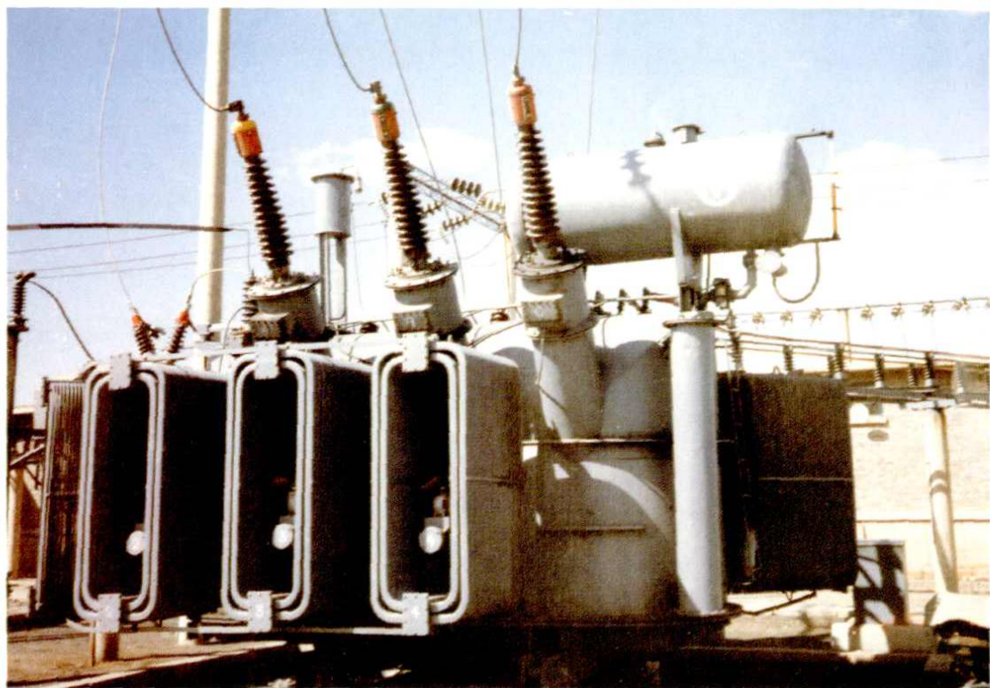
孟县 110 千伏秀水变电站运行中的主变压器
