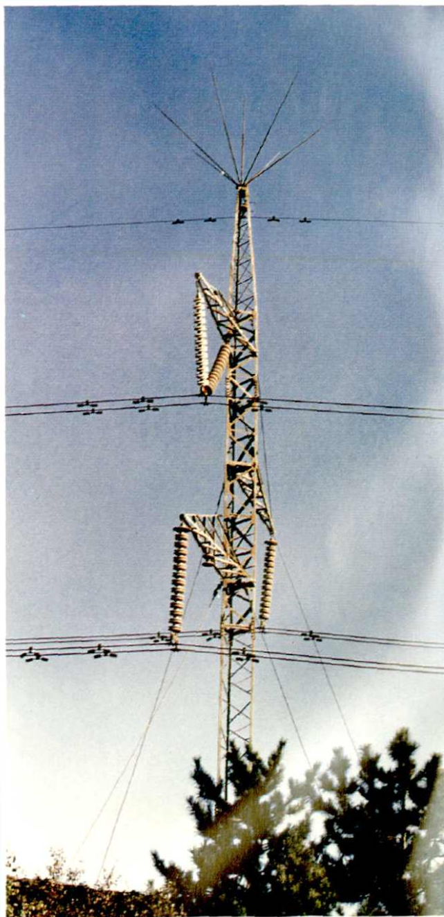
装有消雷器的 220 千伏线路
