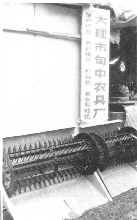
大理市甸中农具厂生产的产品打谷机。
