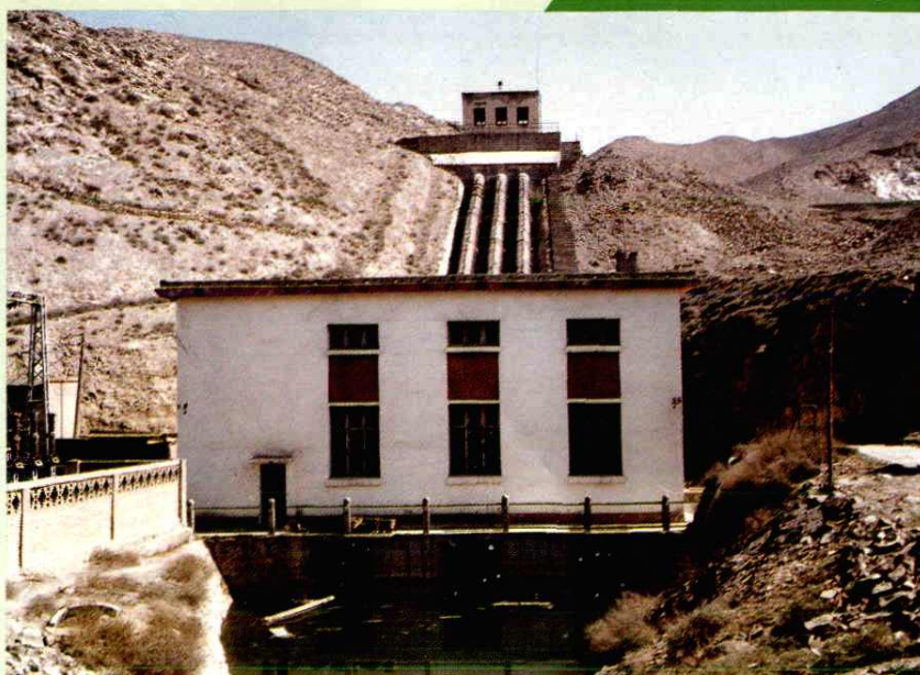
1955年投产的乌拉泊水电站(装机 3 \times 800 千瓦)
