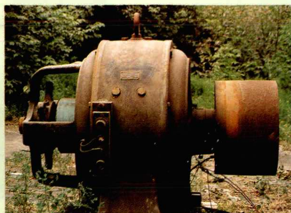
1909年投入运行的皮革厂发电机(75千瓦)
