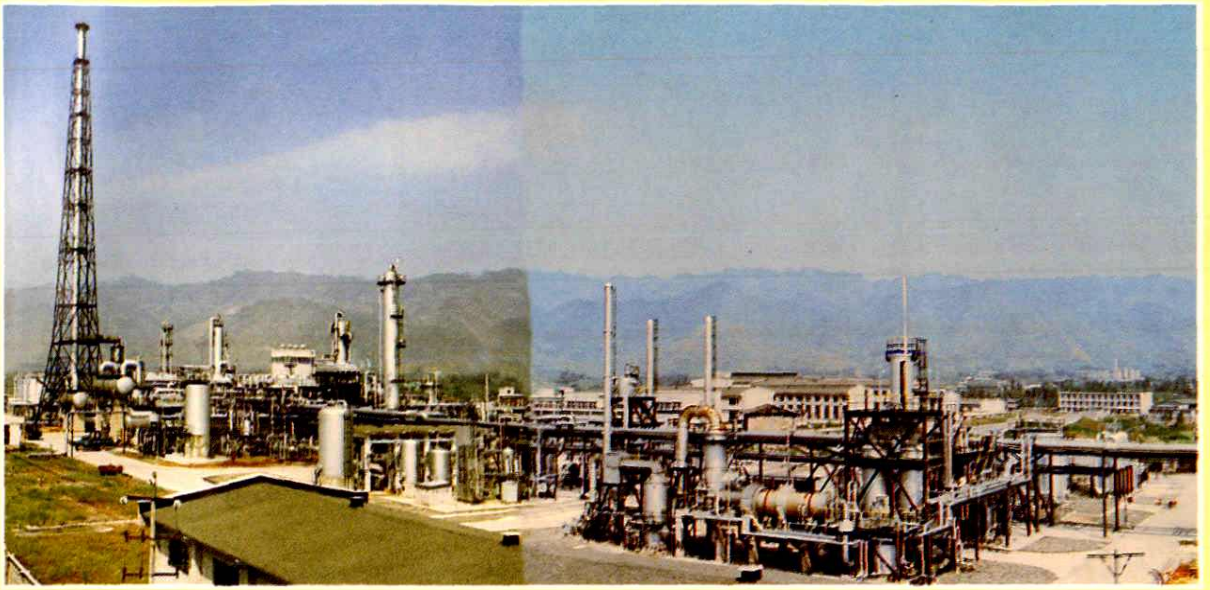
▲ 1979 - 1981年施工建设的川东天然气处理总厂（即卧引工程）全景
