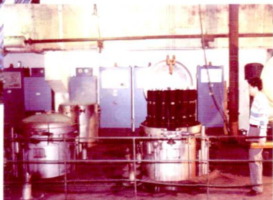
嘉兴第二毛纺织厂条染筒染设备
