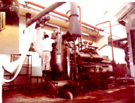
嘉兴第二毛纺织厂溢流染色设备
