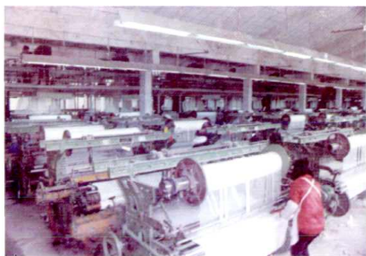
兰溪毛巾总厂毛巾织机
