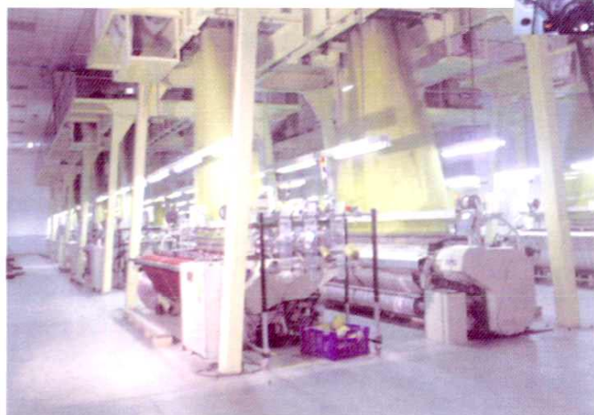
浙江中汇金绫装饰面料公司色织提花剑杆织机
