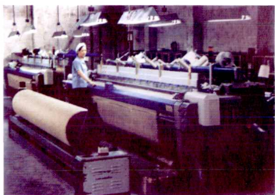
浙江麻纺织厂阔幅剑杆织机
