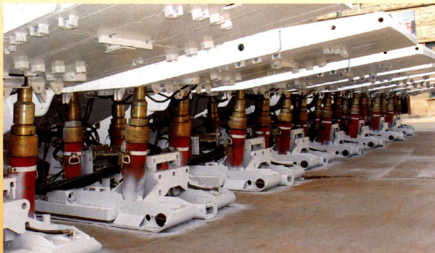
广能集团自主研发的综采液压支架
