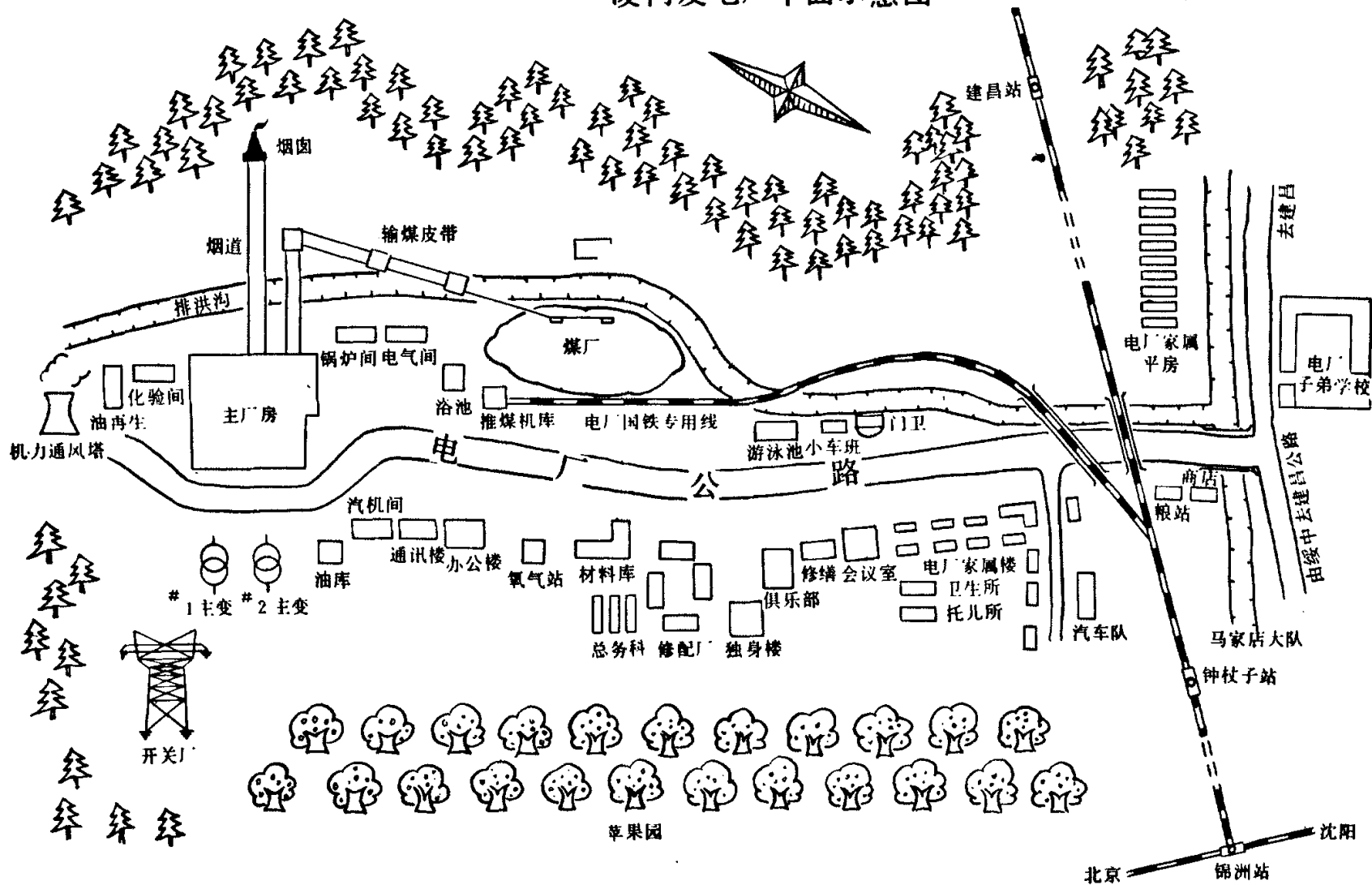
凌河发电厂平面示意图
