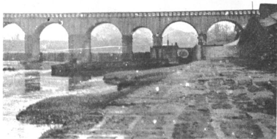
12 大坡乡连拱坝、泵、桥结合工程
