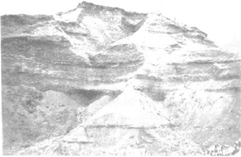
22 遂宁组紫色页岩坡面被雨水切沟浸蚀
