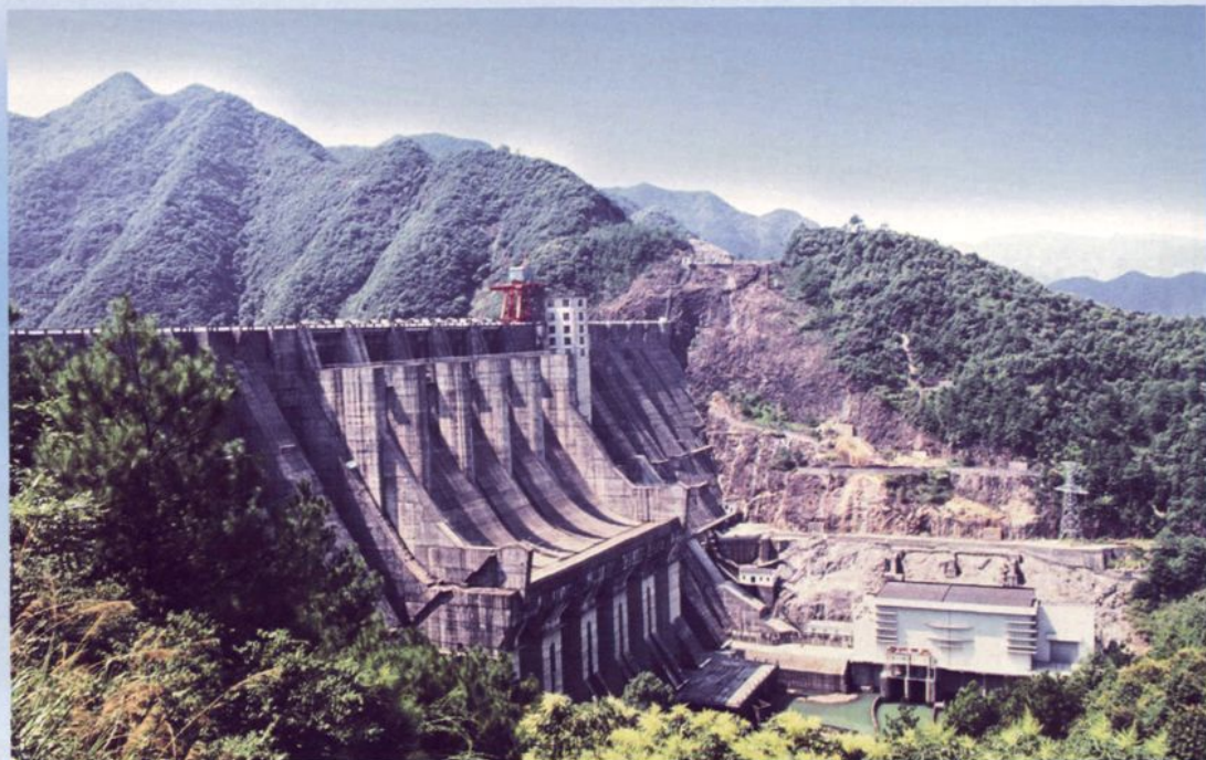
浙江湖南镇水电站
