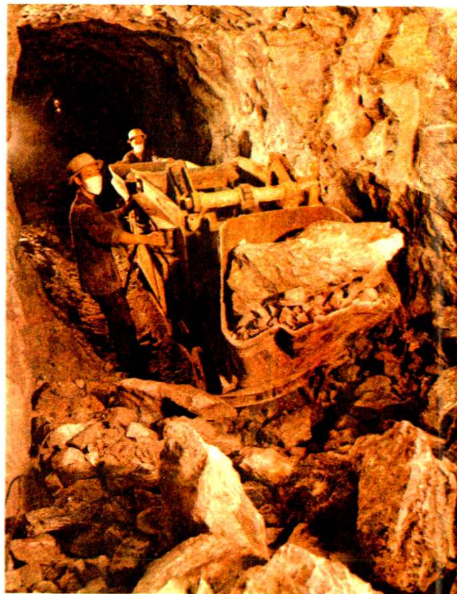
装岩机作业
