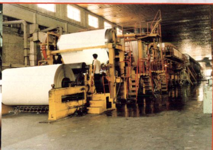
国内第一条涂料白板纸生产线
