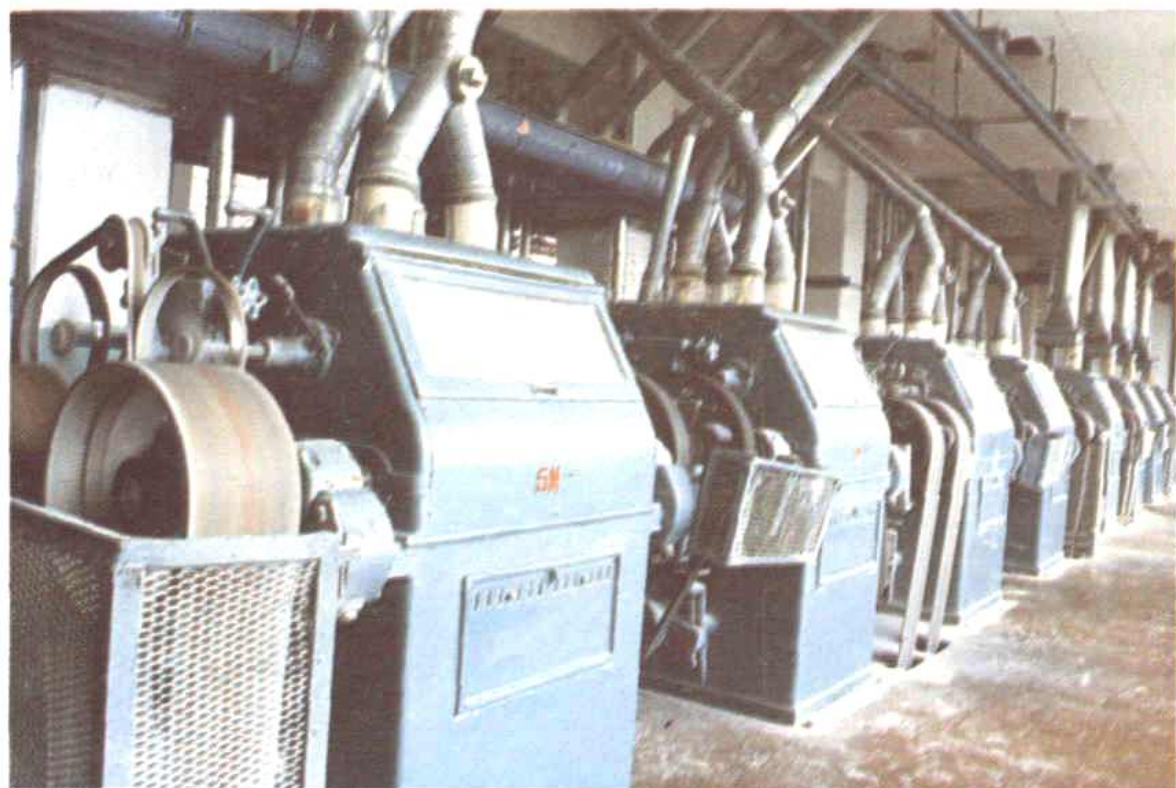
磨粉机
