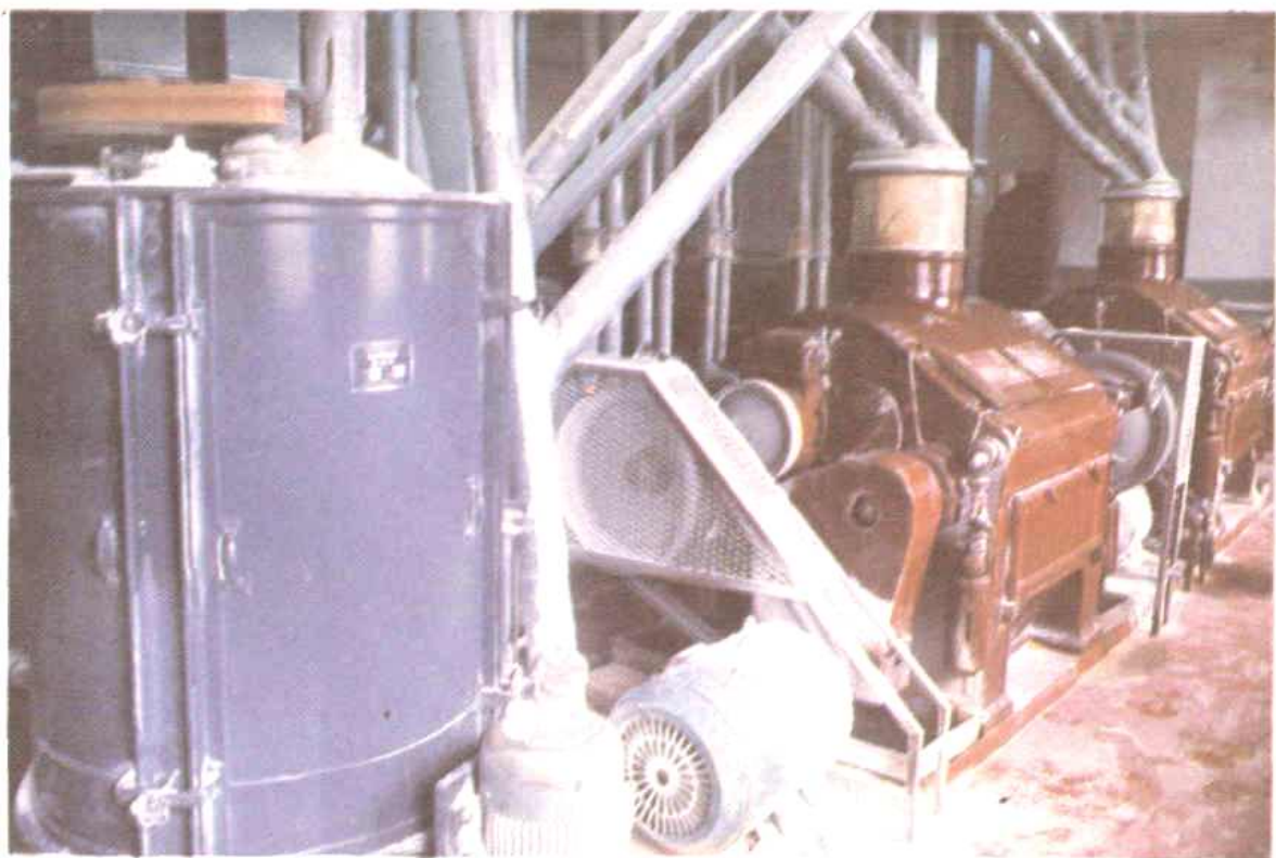
磨粉机
