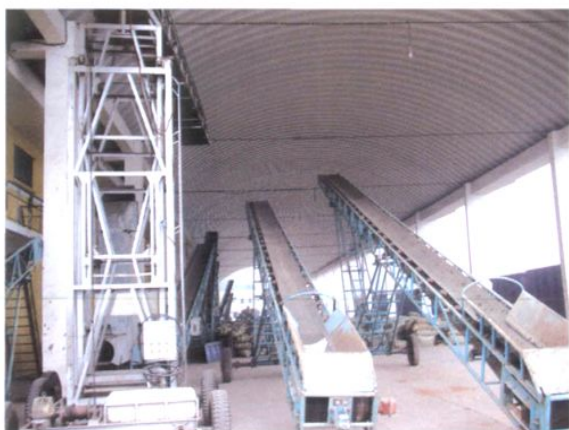
粮仓输送机
