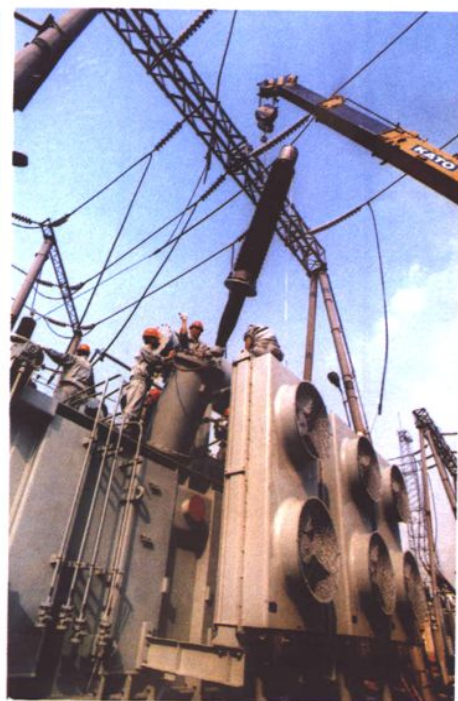
220 千伏五洲变电所变压器安装 (1999 年 7 月摄)
