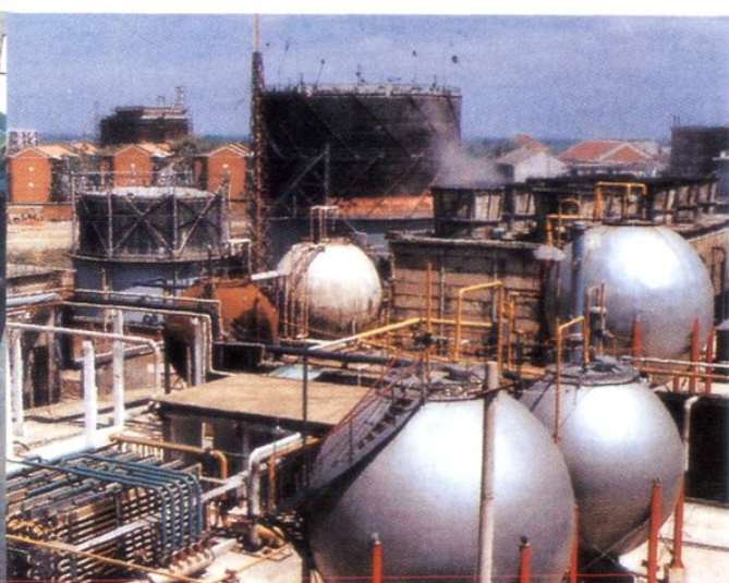
合成氨球罐区
