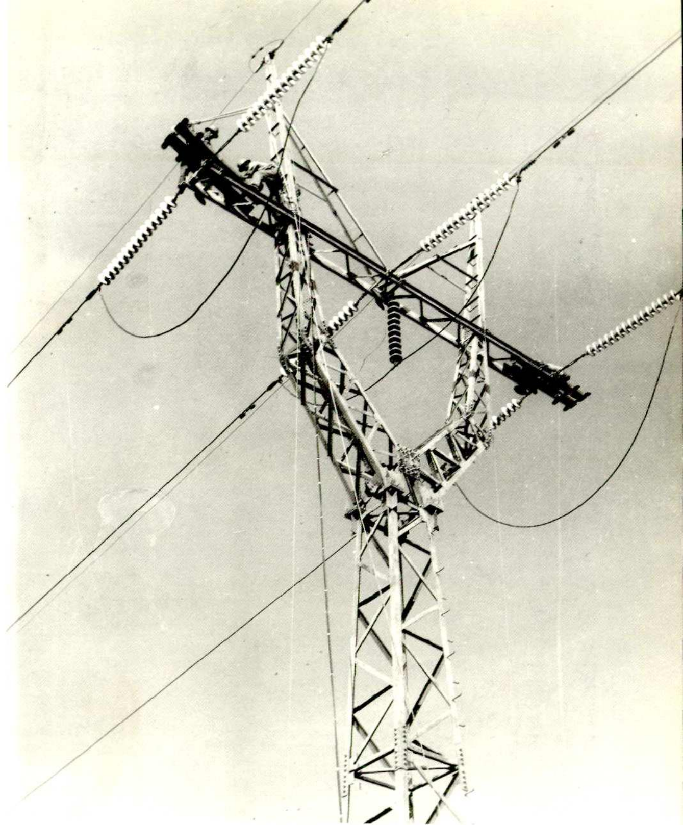
带电作业——加长220千伏横担
