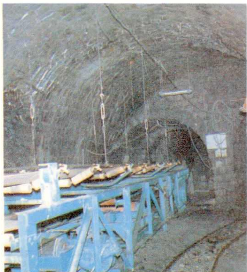
新疆煤矿建设工程处施工安装的艾维尔沟煤矿一九三〇平硐运输巷胶带输送机
