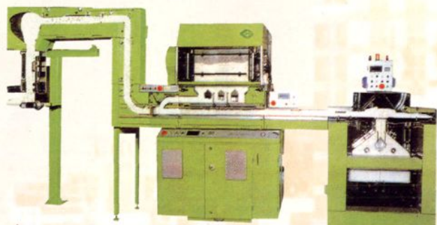
▲ YF12-YB17-YJ35A 型卷烟储存输送装置
