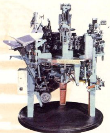
▲ DPXZ-1 型芯柱机
