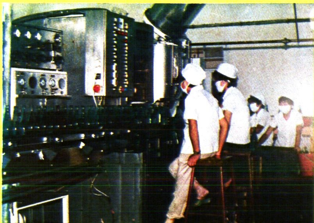
多乐厂饮料灌装流水线
