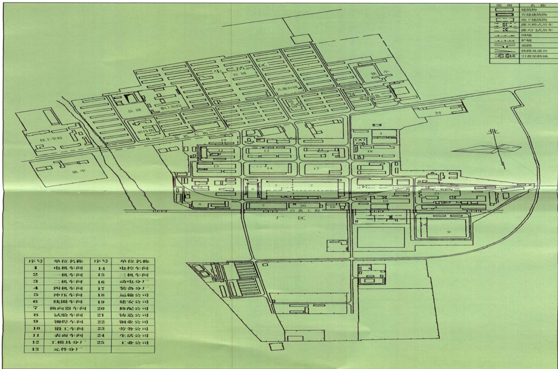
工厂平面图
