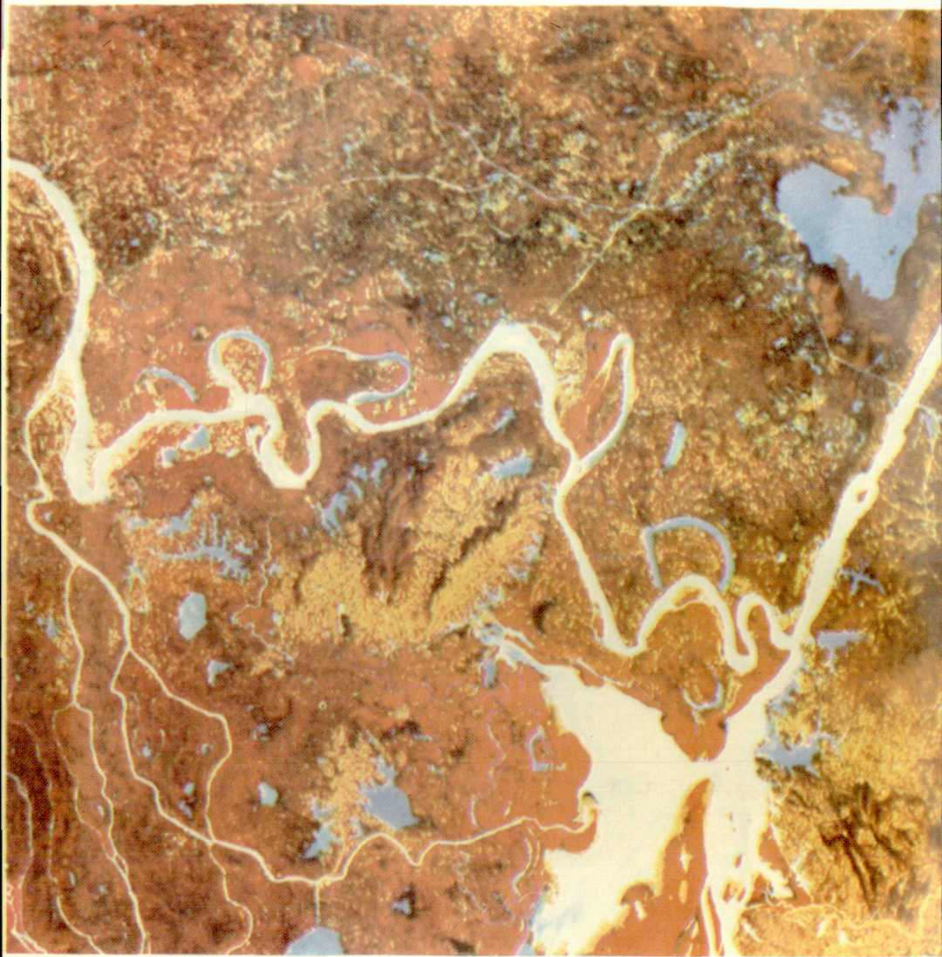
下荆江河道与洞庭湖水系（1980年卫星照片）
