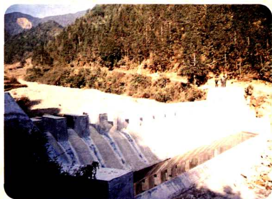
九峰水泥石流防治工程 齿状格栅坝
