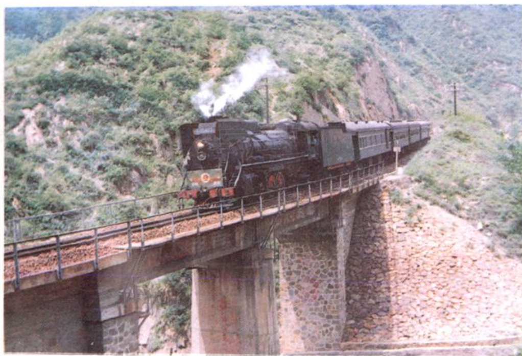
礼垣铁路支线“冶炼厂立交桥”
