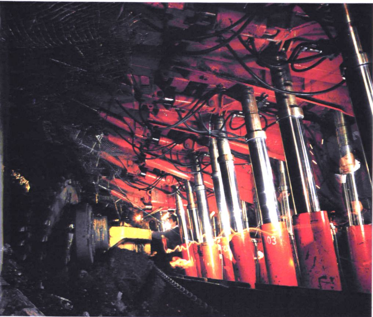
▲ 綜采工作面
