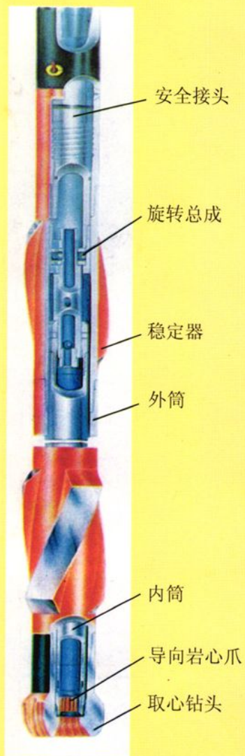
▲ CQX系列常规 取心工具
