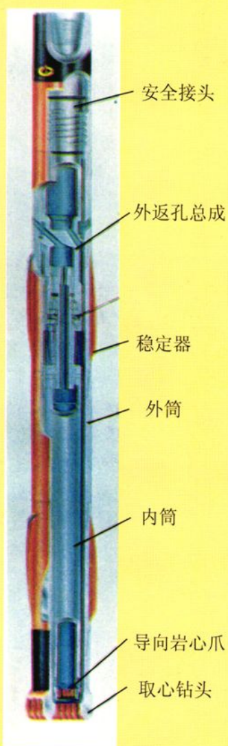
▲ WQX系列外返孔 取心工具
