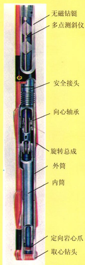
▲ DQX系列定向 取心工具
