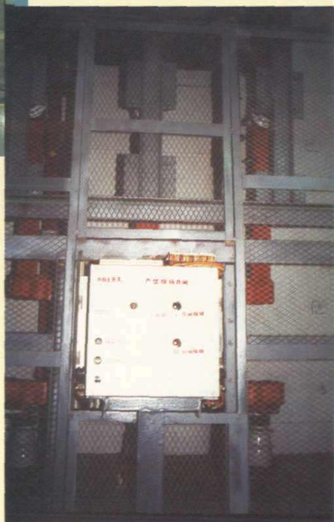
西门子3AH3型真空开关
