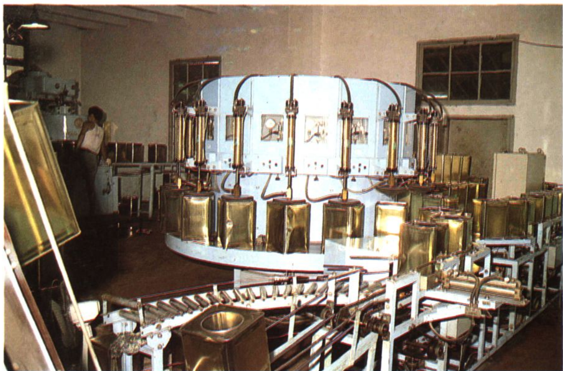
杭州印铁制罐厂18公升罐听全自动流水线
