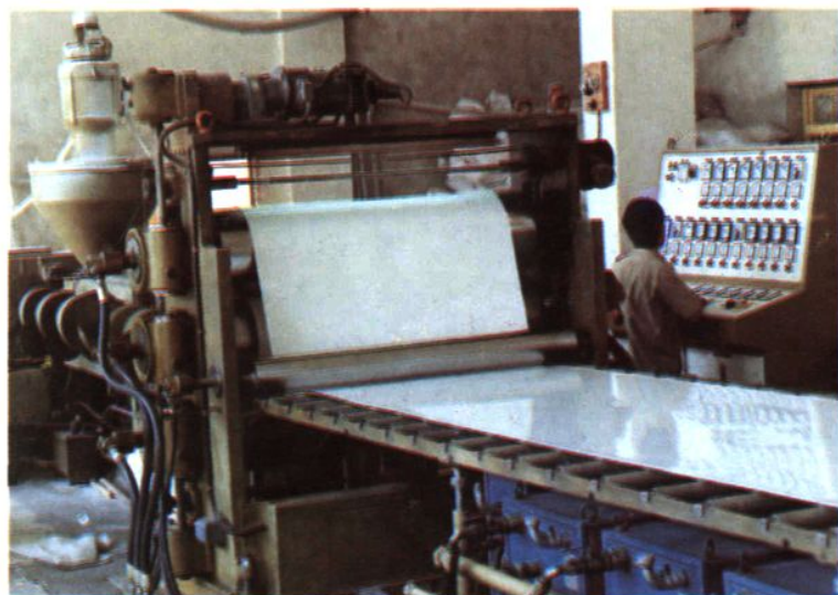
杭州合成塑料总厂ABS 板材生产线
