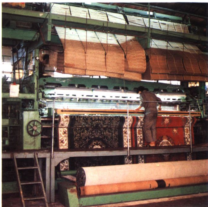
浙江美术地毯厂机 织提花地毯生产设 备
